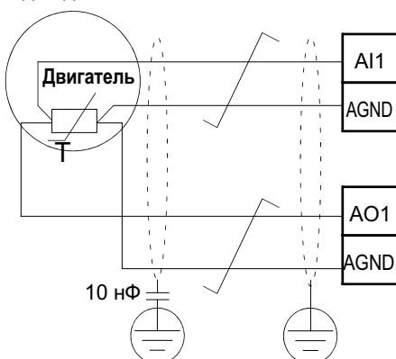
Один датчик
