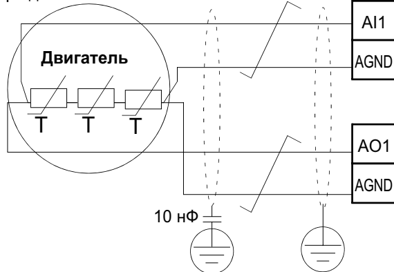
Три датчика
