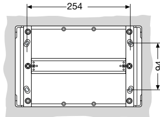
12 модулей
